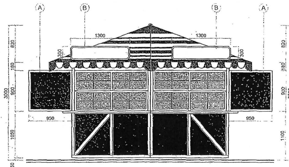
POHĽAD ČELNÝ
