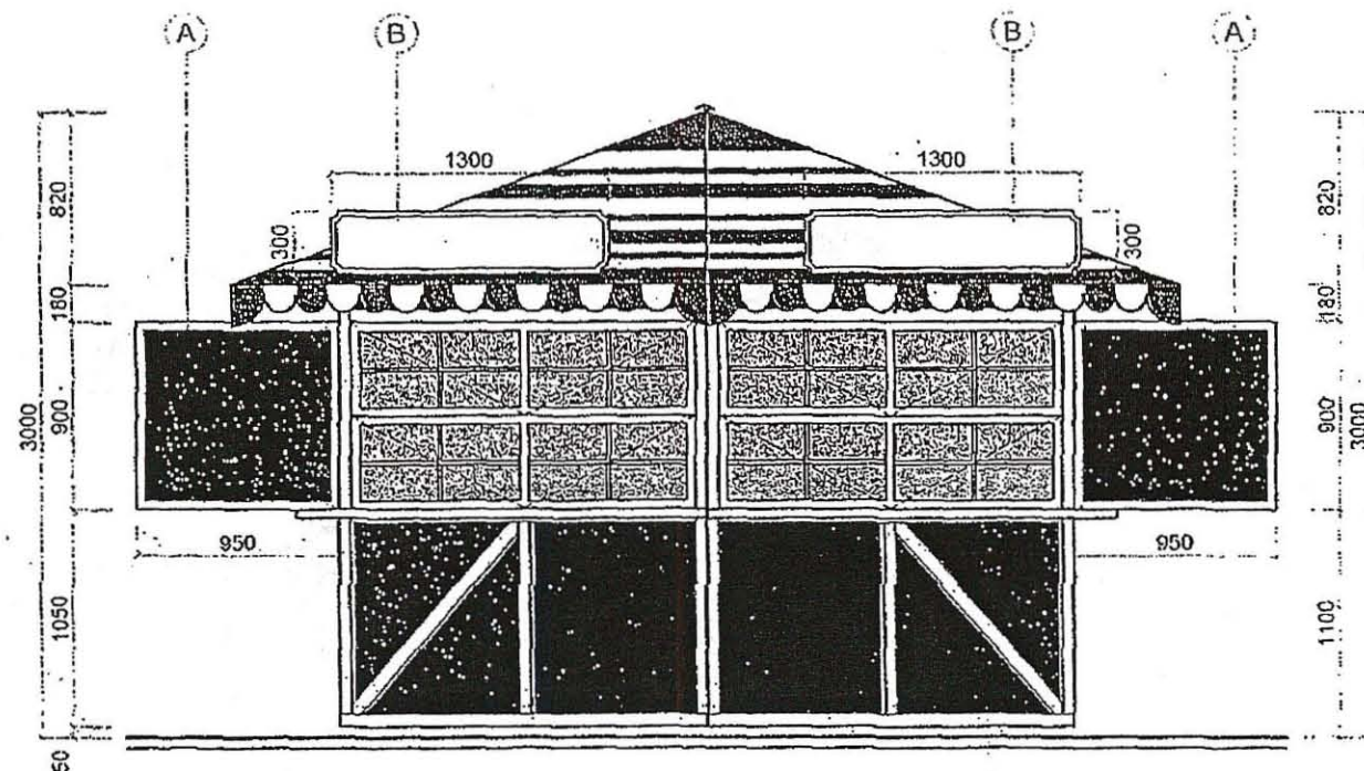
POHĽAD ČELNÝ
