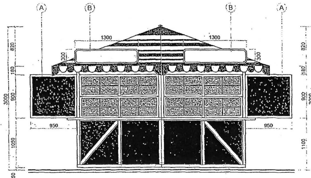
POHĽAD ČELNÝ
