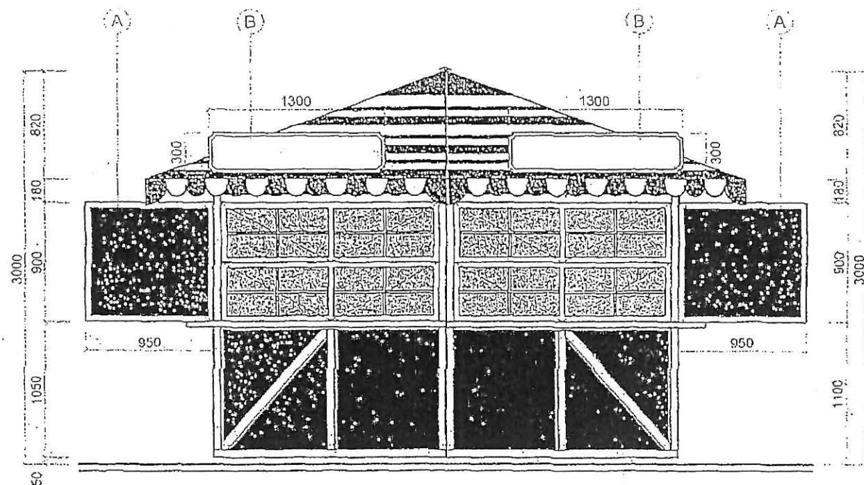
POHLAD ČELNÝ
