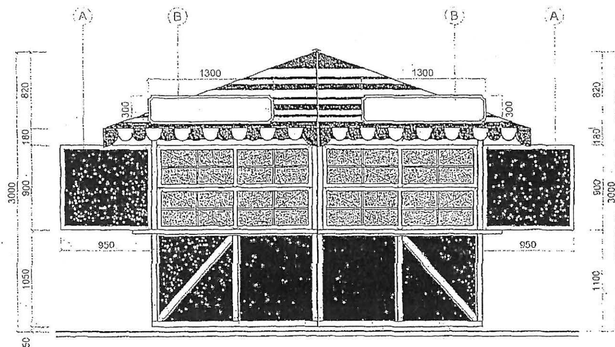
POHLAD ČELNÝ
