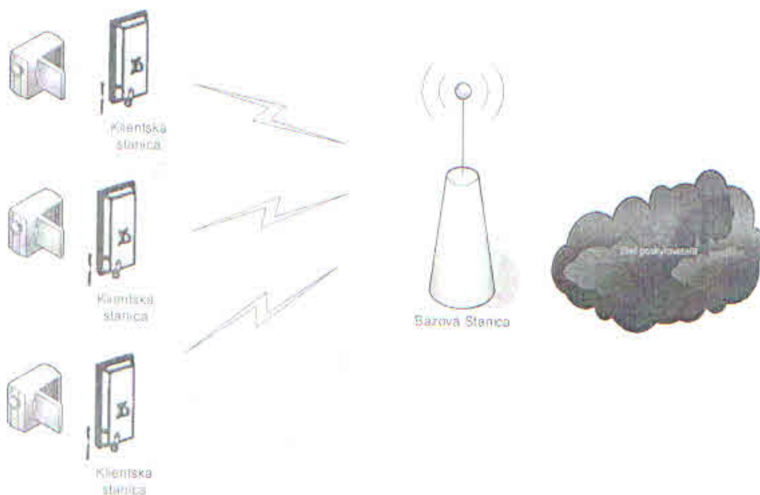
Obrázok 1: Topológia siete
