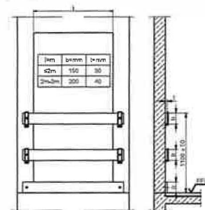
DETAIL OHRADENIA DVERNEHO OTVORU
