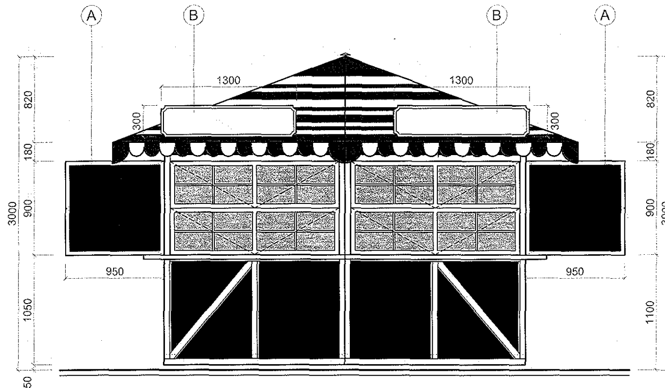
POHĽAD ČELNÝ
