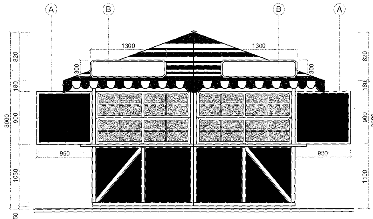
POHĽAD ČELNÝ
