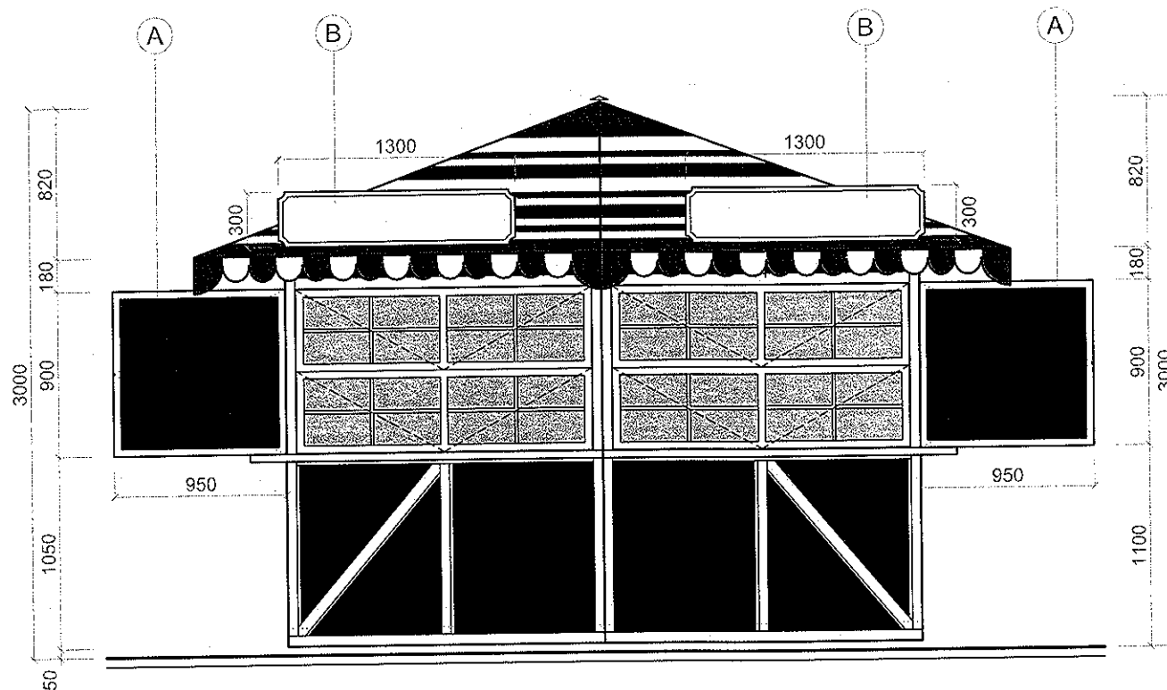
POHĽAD ČELNÝ
