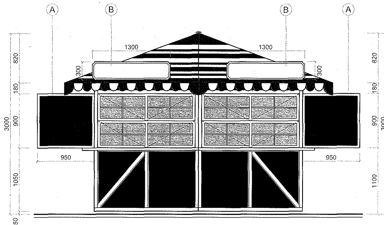
POHĽAD ČELNÝ
