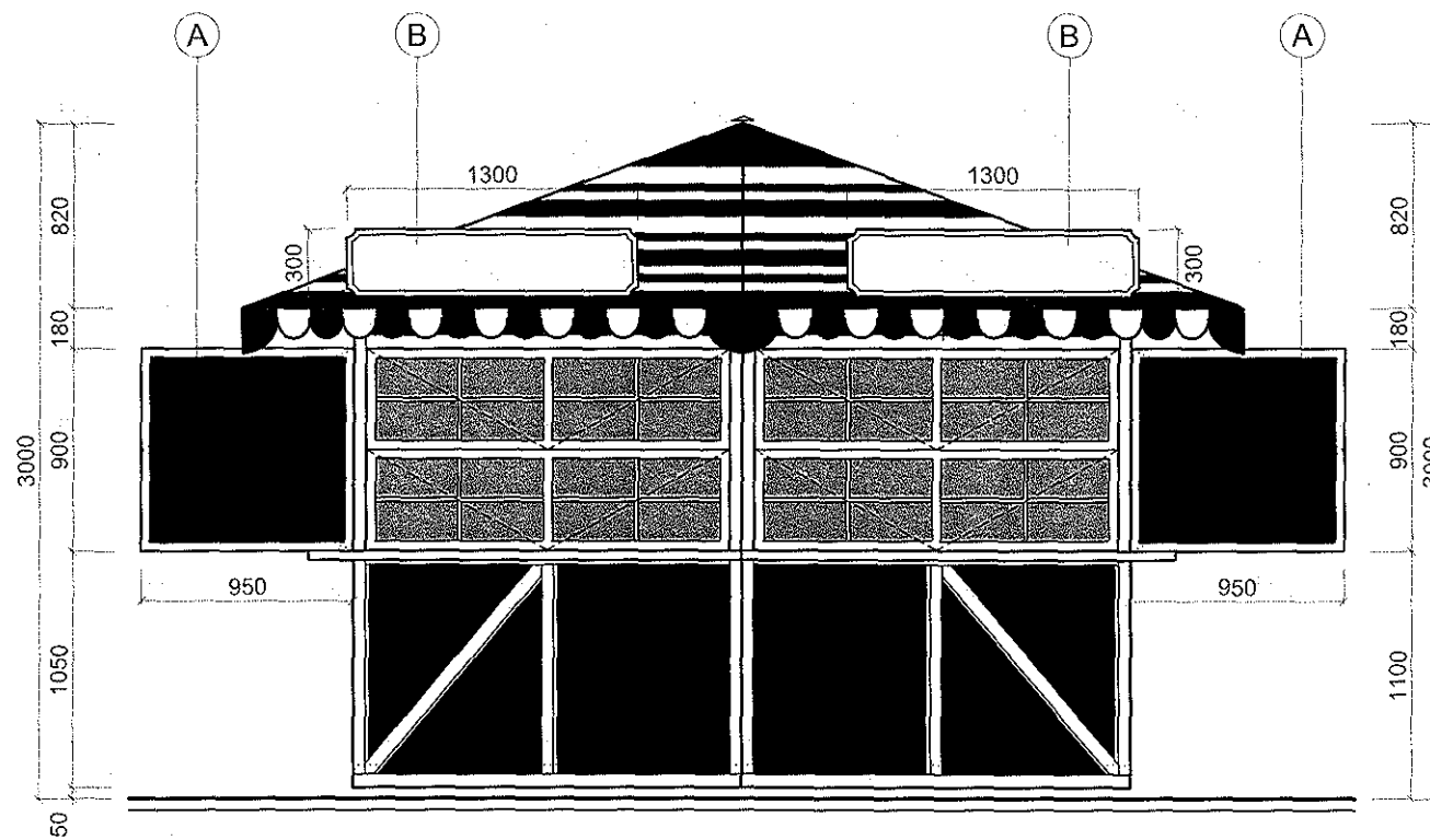
POHLAD ČELNÝ
