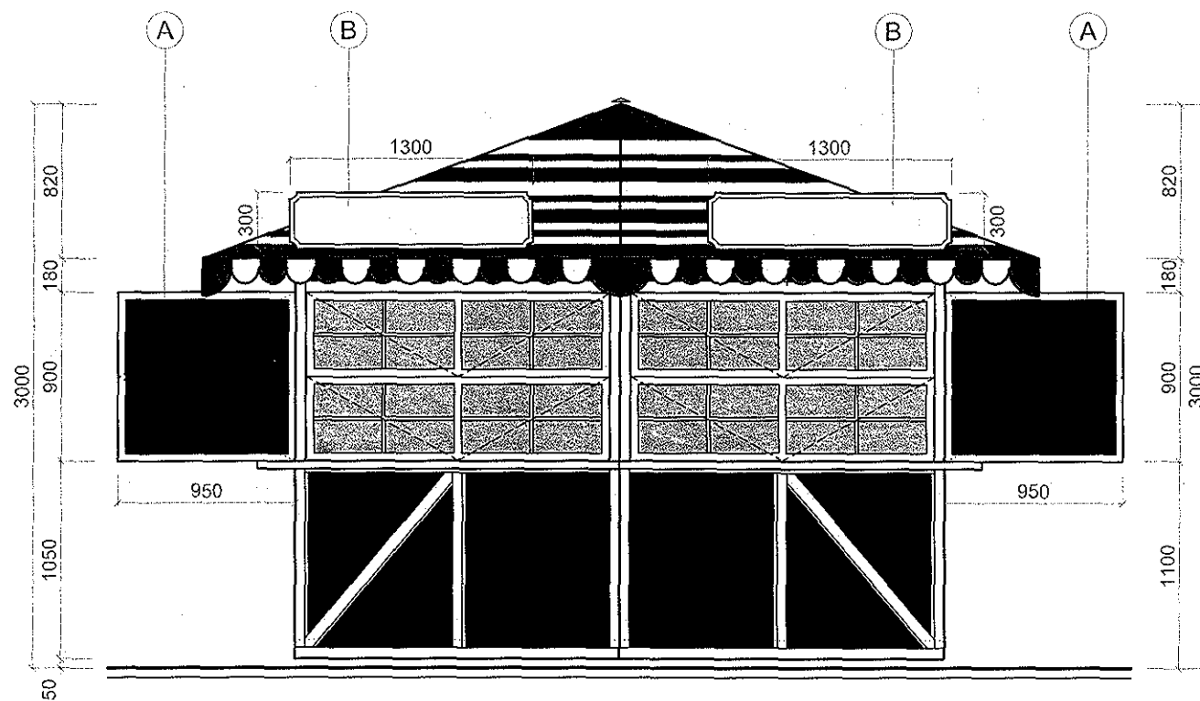
POHĽAD ČELNÝ
