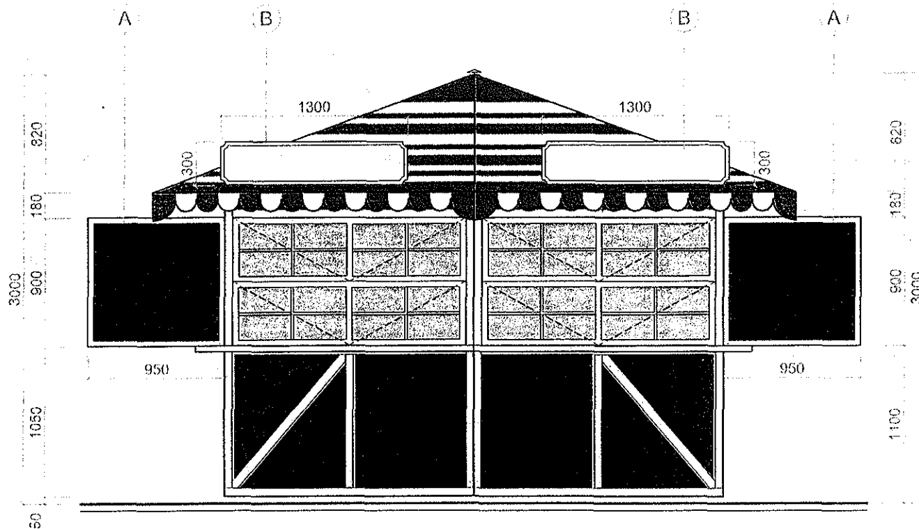
POHĽAD ČELNÝ
