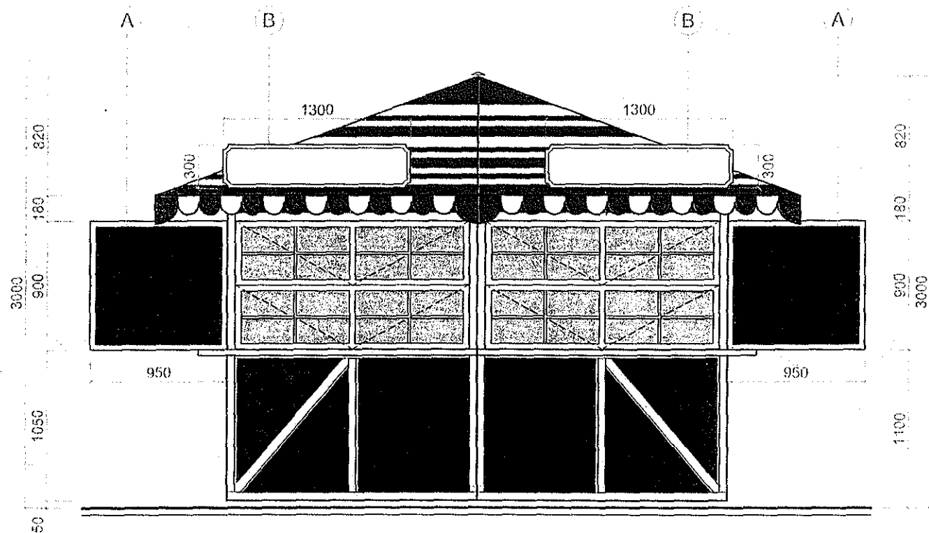
POHĽAD ČELNÝ
