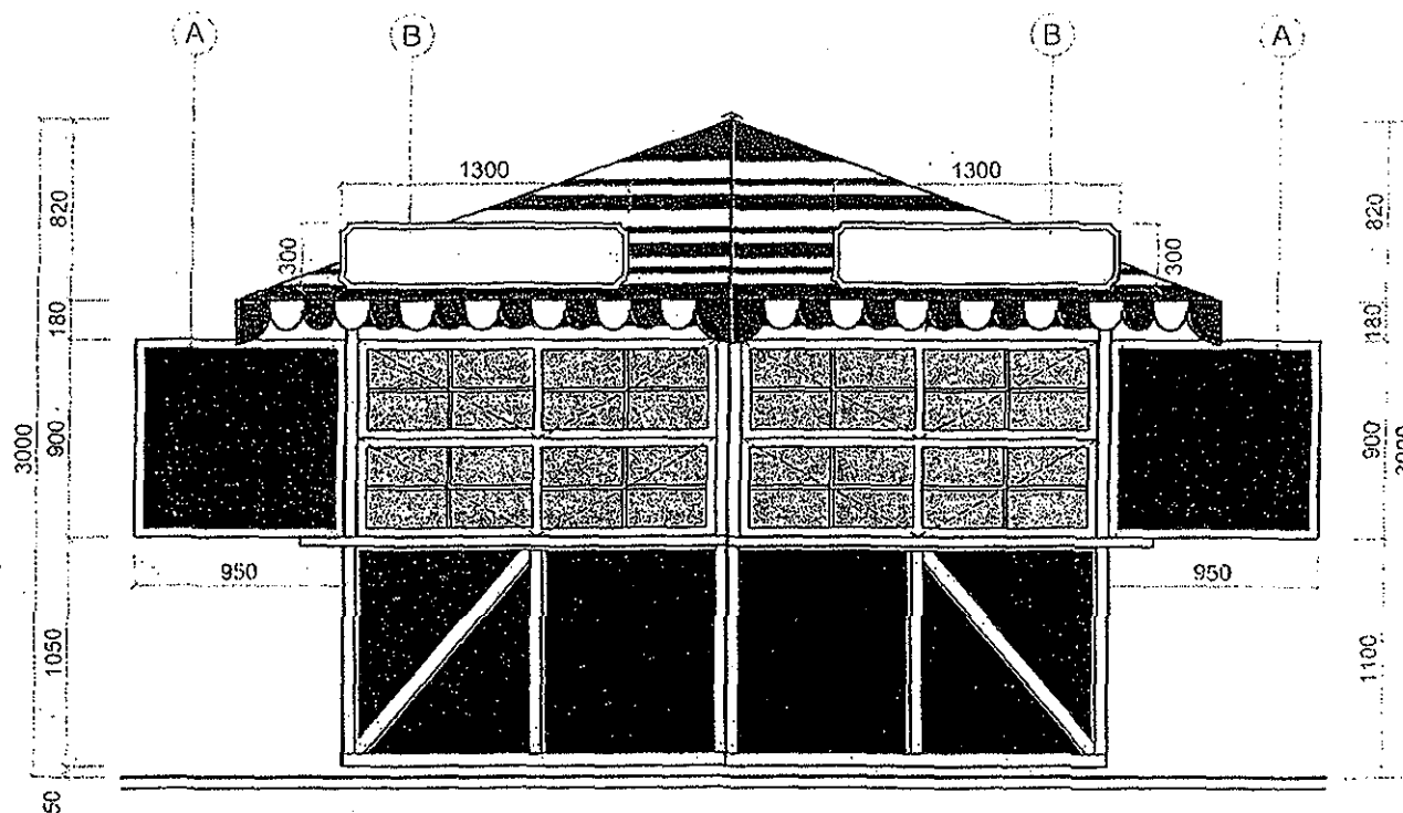
POHĽAD ČELNÝ
