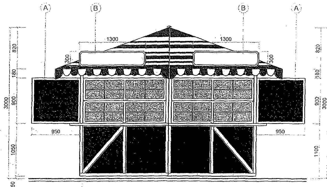
POHĽAD ČELNÝ
