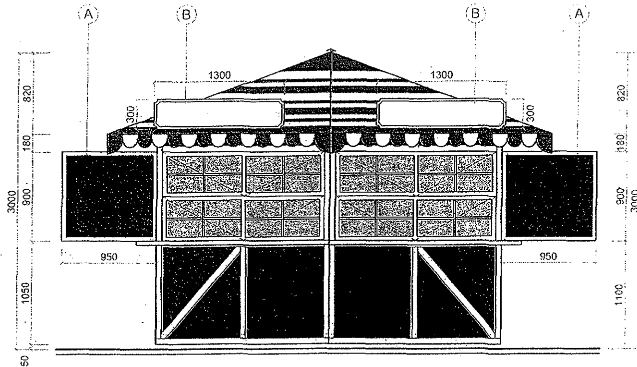
POHLAD ČELNÝ
