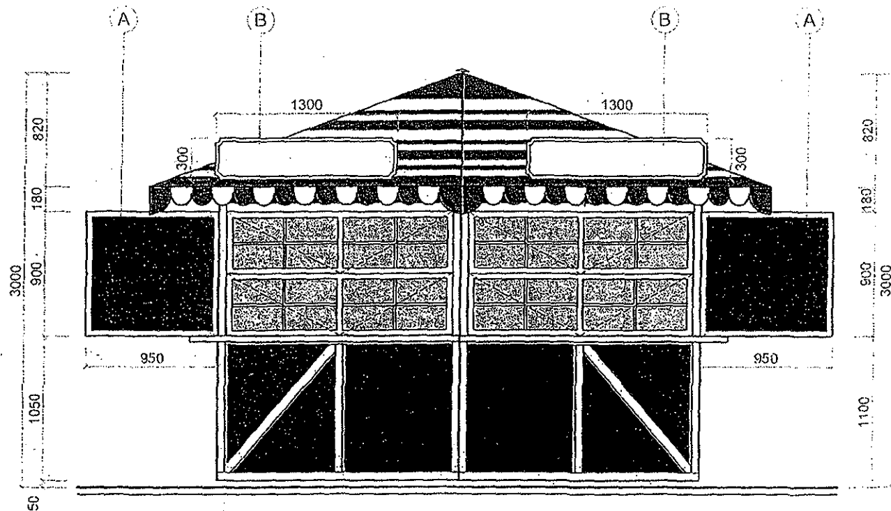
POHLAD ČELNÝ
