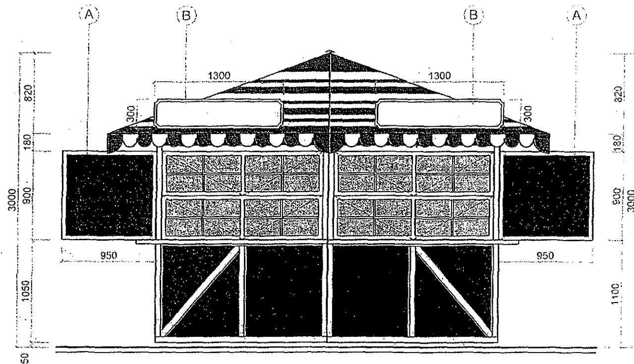
POHĽAD ČELNÝ
