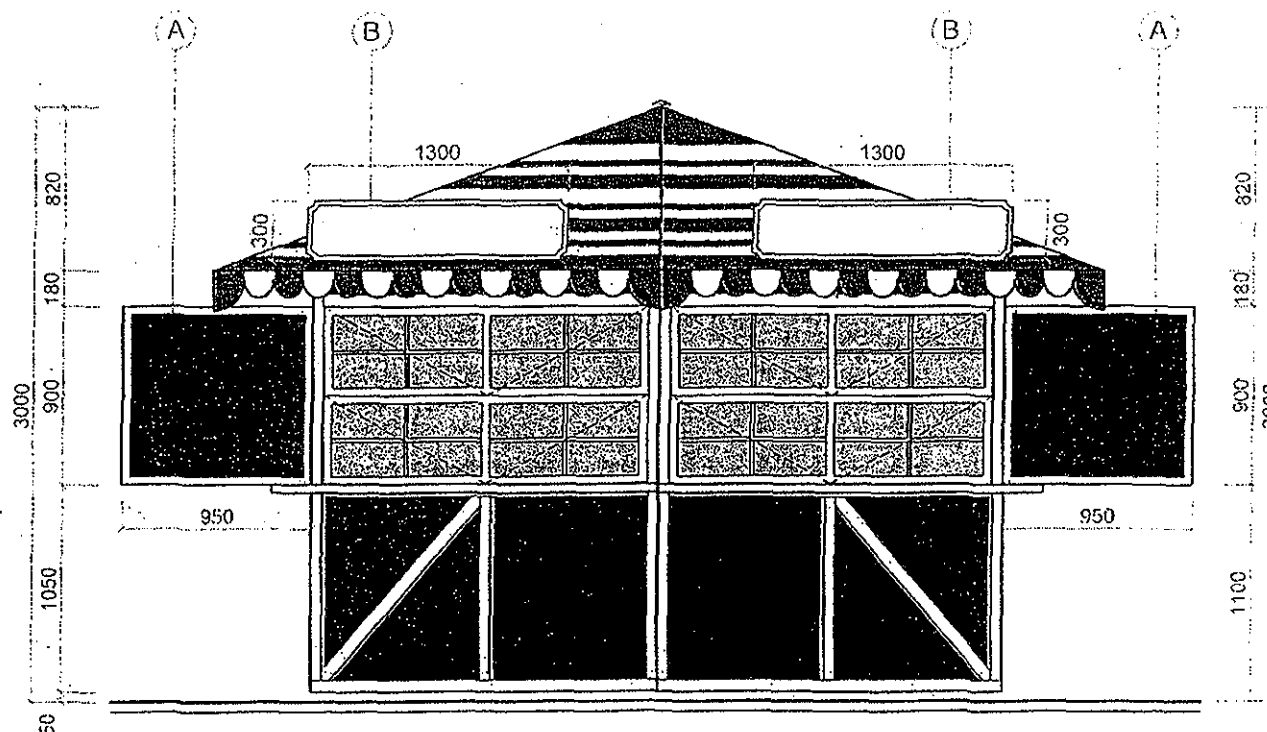
POHĽAD ČELNÝ
