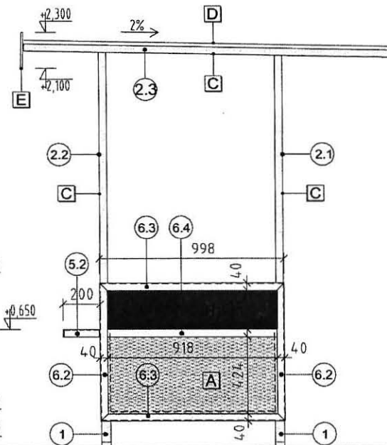
POHĽAD BOČNÝ, M 1:20
