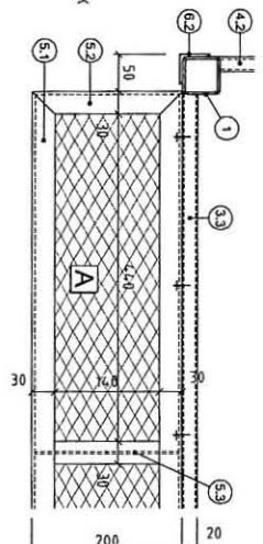
DETAIL 2 - NAROŽIE ODKLADACIEHO PULTU, M 1:1
