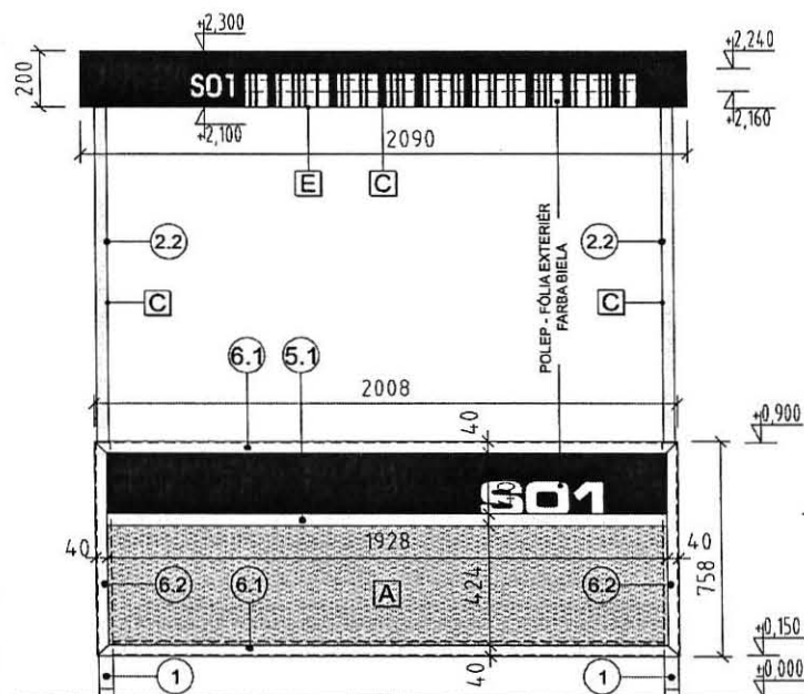
POHĽAD PREDNÝ, M 1:20
