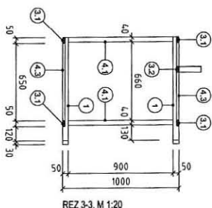
REZ 3-3. M 1:20
