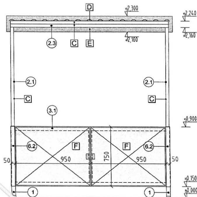
POHĽAD PREDNÝ, M 1:20
